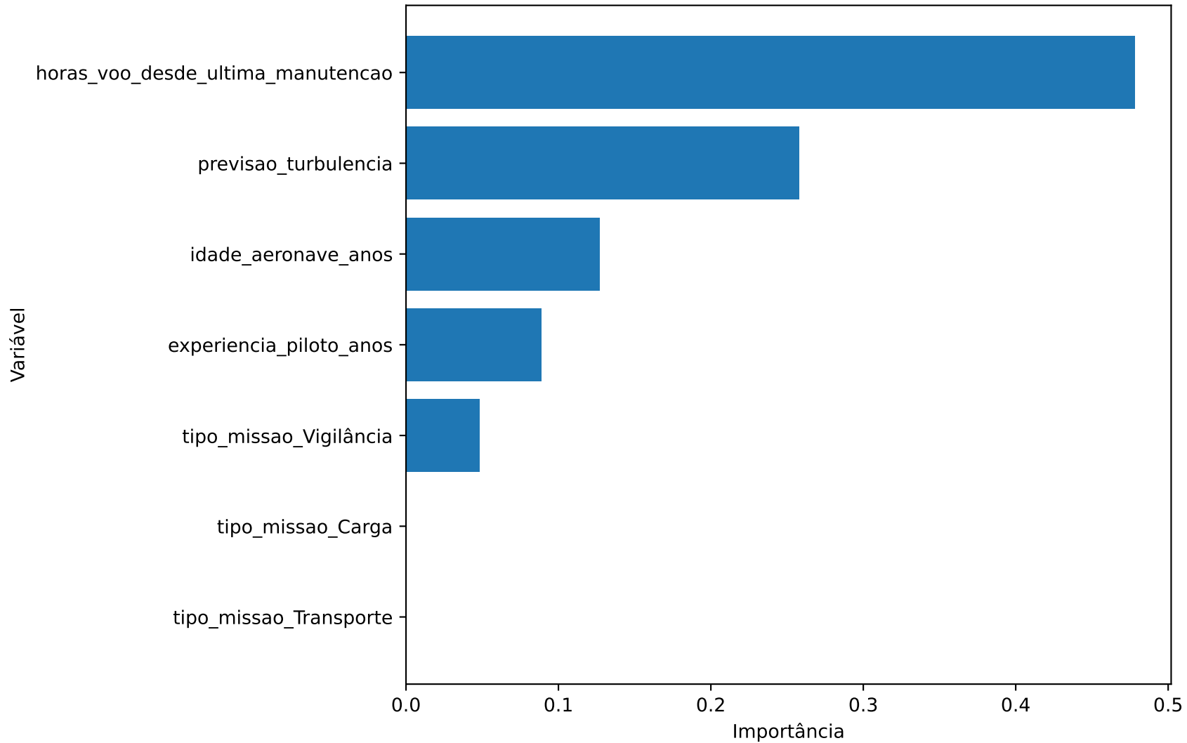
Top variáveis mais importantes — xgboost
